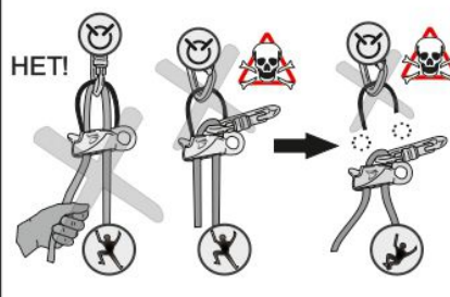
Рис. 16. Спуск по веревке
